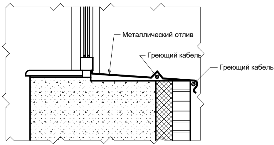
Узел 1. Обогреваемый отлив
