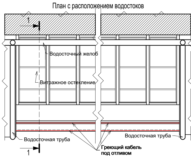
Узел 1. Обогреваемый отлив
