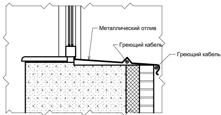
Узел 1. Обогреваемый отлив
